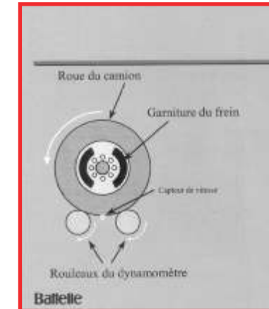
Les freinomètres à rouleaux
